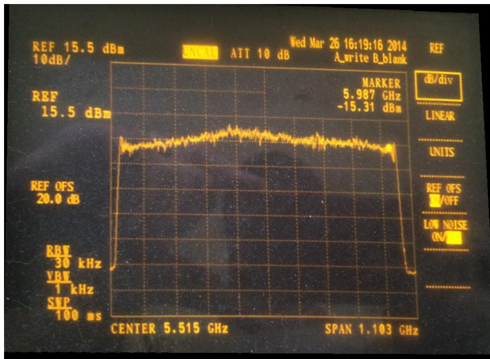
Spectre du brouillage de 5 à 6 GHz
